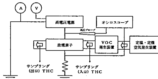
図2 試験装置概要
