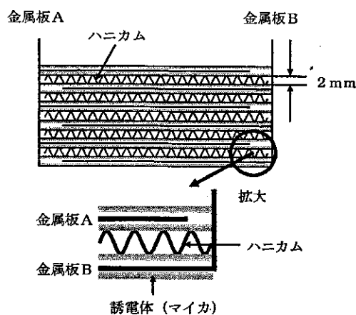
図1 プラズマ発生部(放電素子)
