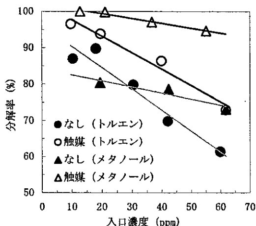
図4 トルエン、メタノール分解における触媒の効果 吸着剤: 疎水性ゼオライト
